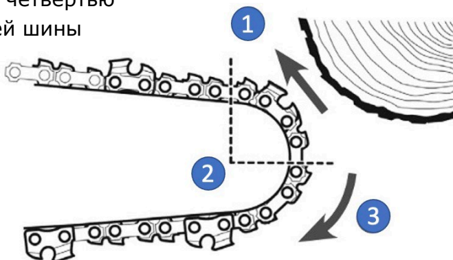
Рис. Отскок или вниз и назад на оператора 1. Направление отскока 2. Зона опасности возникновения отдачи 3. Направление движение цепи
